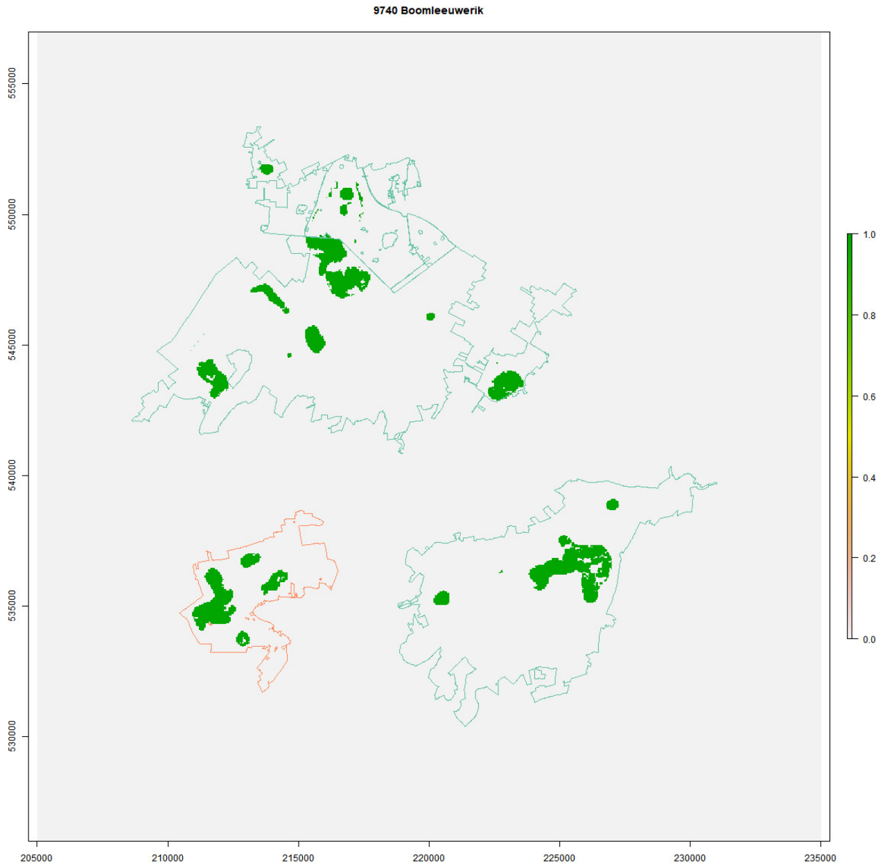
Figuur 2.3. Kwantielkaart van Boomleeuwerik. Afgebeeld is het kleinste gebied waar 50% van de populatie zich bevindt (q50-kaart).
